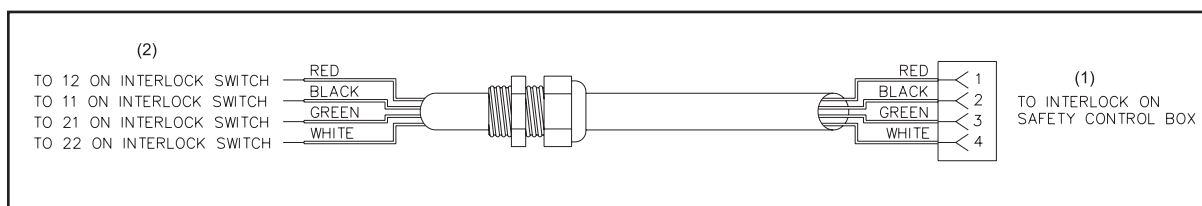
47-142862-000 - Door Interlock Switch Cable Assembly
